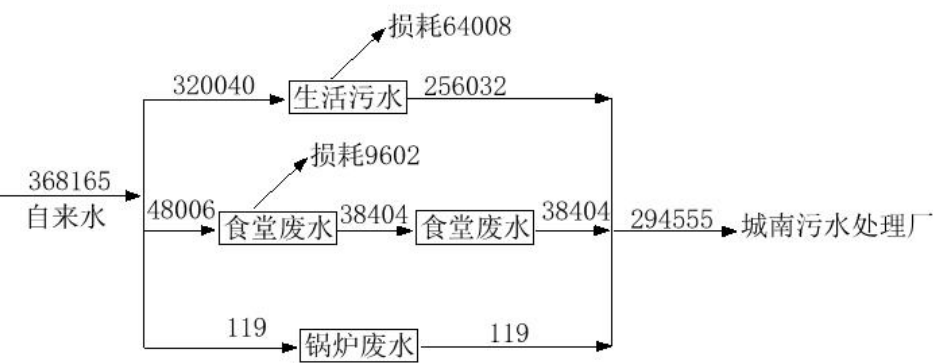
图 2-1 技改前全厂水平衡图 (t/a)
