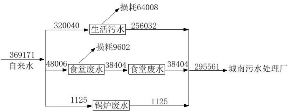
图 2-2 技改后全厂水平衡图 (t/a)
